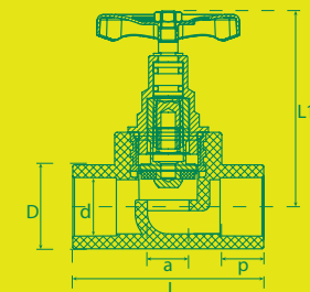
Dimensiones de Válvulas de Globo PP-R
