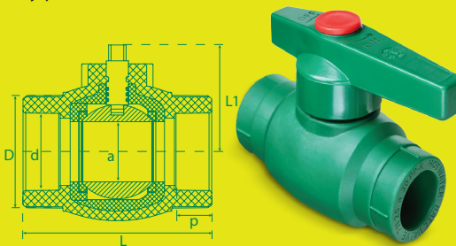
Dimensiones de Válvulas de Esfera PP-R
